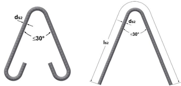
Bijlegwapening voor hijsen (trek)
