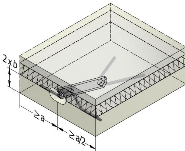
Sandwichplaatanker SA-SP - Draagvermogen, installatieafmetingen
