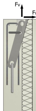
Sandwichplaatanker SA-SP - Draagvermogen, installatieafmetingen
